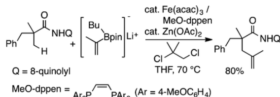
図5 亜鉛化合物を鍵中間体とした二置換インドール合成, および鉄触媒による sp 3 C-H 結合の活性化
